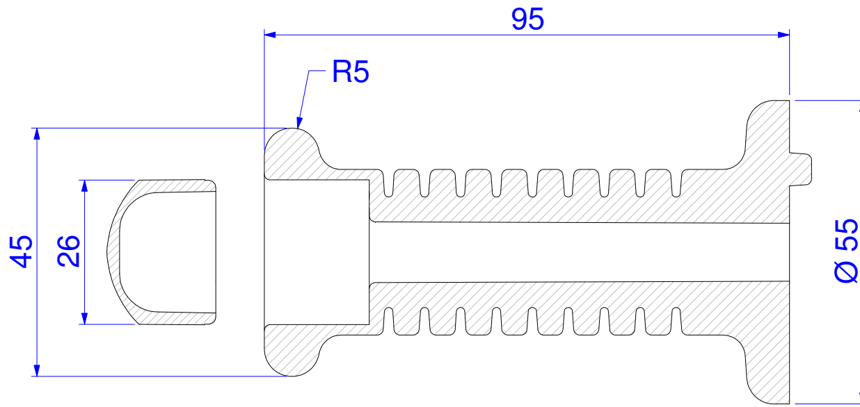
SEZIONE C-C 1:1
